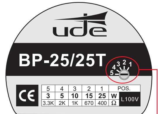
SELECTOR ROTATIVO DE POTENCIAS SÉLECTEUR ROTATIF DE PUISSANCES ROTARY SWITCH
