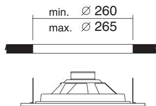
MONTAJE EN FALSO TECHO MONTAGE DANS FAUX PLAFOND FALSE CEILING ASSEMBLY
